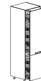
A14-60-207 výsuvná (600 x 565 x 2070)
